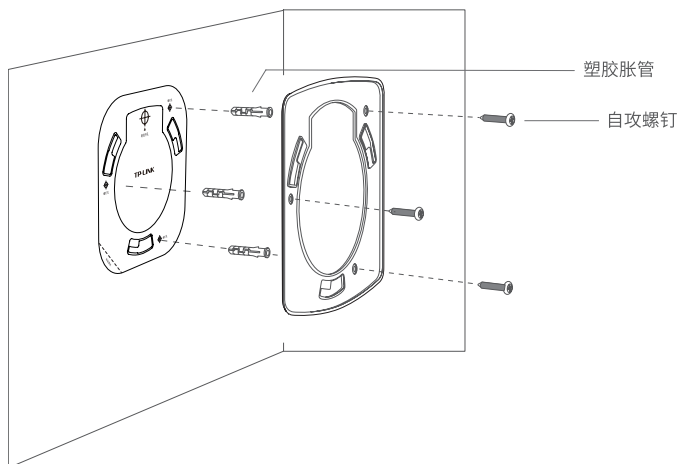
图3-11 固定安装架到墙面示意图
